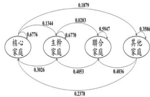
圖 3：「經濟狀況高」的馬可夫鏈
