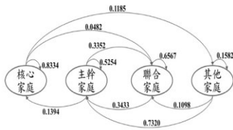
圖 2：「經濟狀況中」的馬可夫鏈
