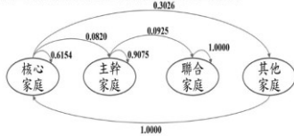
圖 1：「經濟狀況低」的馬可夫鏈
